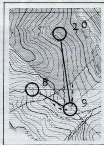
A conformação do terreno evitando o ângulo agudo
